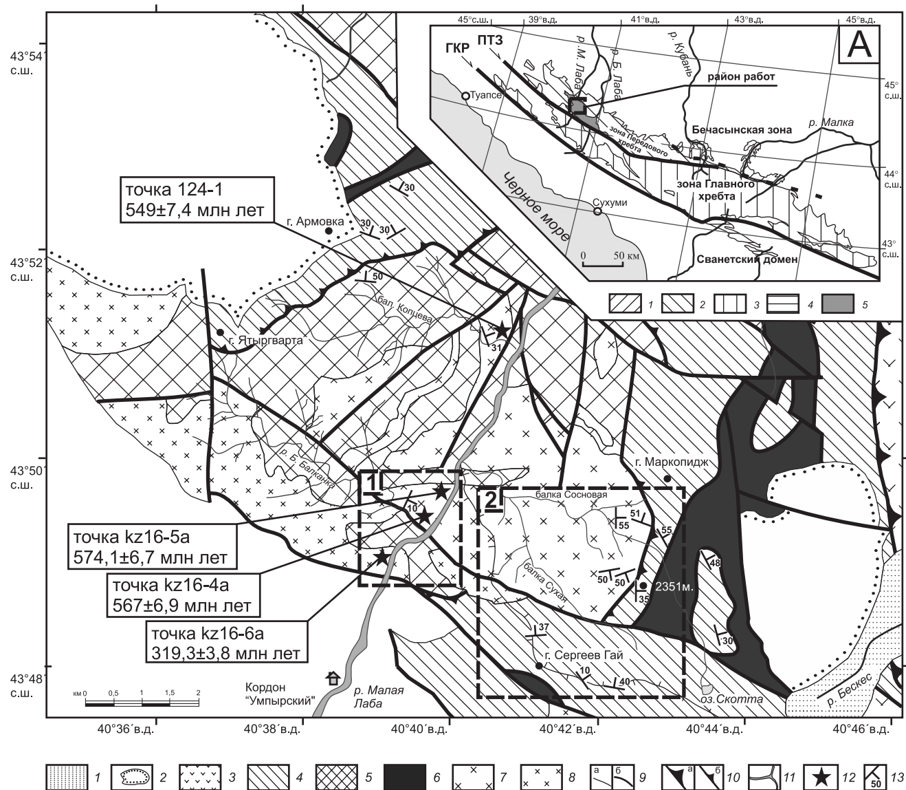
Рис. 1. Схема тектонического строения Блыбского метаморфического комплекса в бассейне реки Малая Лаба. Цифры 1, 2 на рисунке — детально изученные участки. 1 — четвертичные образования; 2 — юрские осадочные отложения; 3 — отложения урупского вулканогенно-осадочного комплекса; 4 — армовские метаморфиты; 5 — балканская свита; 6 — гипербазиты; 7 — Балканский массив кварцевых метадiorитов; 8 — гранодиориты Южной интрузии; 9 — геологические границы: а — стратиграфические, б — тектонические; 10 — границы покровов: а — Урупского, б — Армовского; 11 — речная сеть; 12 — места отбора геохронологических проб (В сносах даны номера точек и соответствующие возрасты); 13 — ориентировки плоскостных текстур. Во врезке А: схема тектонического районирования доюрского основания Большого Кавказа. Сокращения: ГКР — Главный Кавказский разлом; ПТЗ — Пшекиш-Тырныаузская зона. 1 — Бечасынская зона; 2 — зона Передового хребта; 3 — зона Главного хребта; 4 — выходы пород Дизской серии; 5 — Блыбский метаморфический комплекс.
