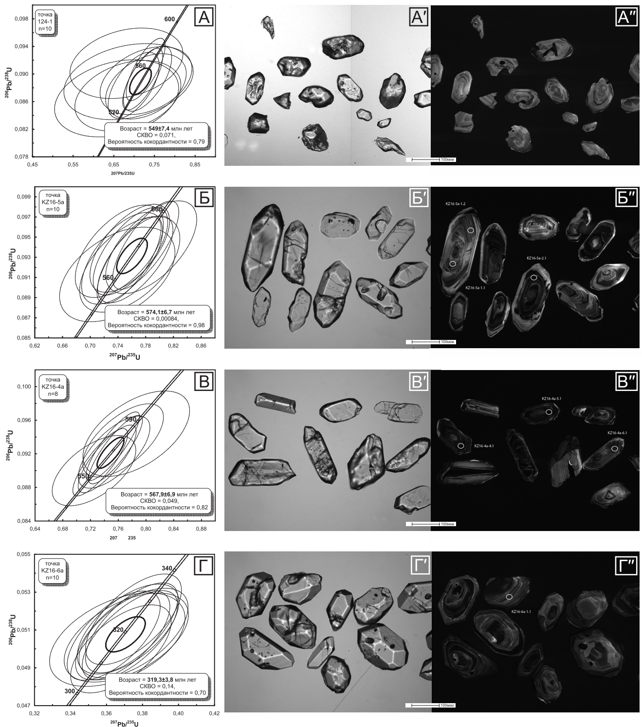
Рис. 2. Конкордии исследованных цирконов, а также их оптические и катодолюминисцентные изображения. А, А', А'' — Балканский массив (северная оконечность, балка Копцева, точка 124-1); Б, Б', Б'' — Балканский массив, район балки Сухая, точка kz16-5a); В, В', В'' — Балканский массив (южная оконечность, р. Бол. Балканка, точка kz16-4a). Г, Г', Г'' — Южная интрузия гранодиоритов (точка kz16-6a). Эллипсы ошибок измерений возраста имеют доверительные интервалы 2σ.
