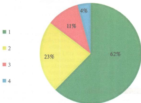
Рис. 1. Распределение видов ценофлоры сосновых лесов Дагестана по отношению к увлажнению почвы. 1 – мезофиты, 2 – мезоксерофиты, 3 – ксерофиты, 4 – ксеромезофиты.
