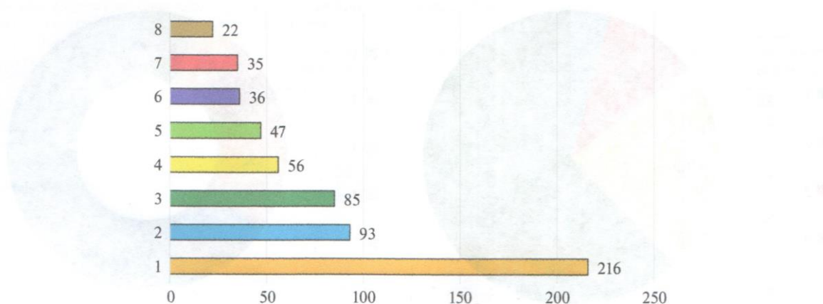
Рис. 3. Соотношение видов в ценофлоре сосновых лесов Дагестана по флороценотипам.
